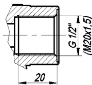
Рисунок Б.12 – Чертеж средств взрывозащиты (компактное исполнение, тип присоединения к процессу «зондовый с лубризатором»)
