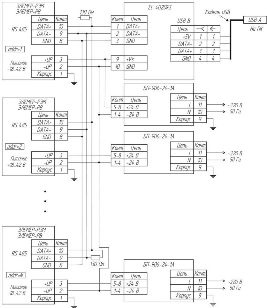
Рисунок А.8 – Схема электрическая подключений ЭЛЕМЕНТ-РВ с протоколом обмена ModBus в сеть
