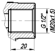
Рисунок Б.10 – Чертеж средств взрывозащиты (компактное исполнение, тип присоединения к процессу «зондовый»)
